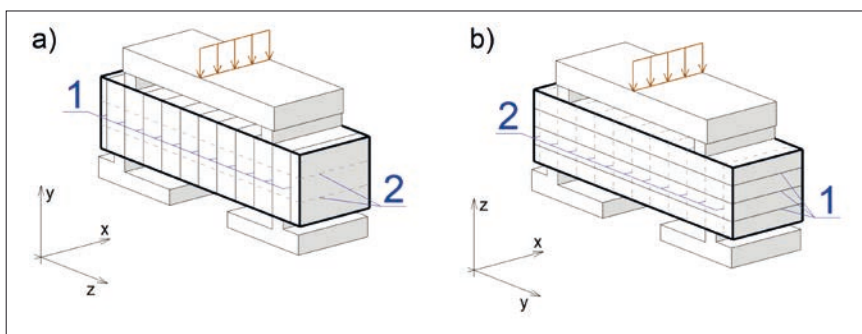
Rys. 8. Schemat obciążenia w badaniu wytrzymałości na ścinanie powierzchni międzywarstwowej: a) obciążenie wzdłuż osi Y, b) obciążenie wzdłuż osi Z (1 – połączenie międzywarstwowe, 2 – połączenie międzypasmowe)
