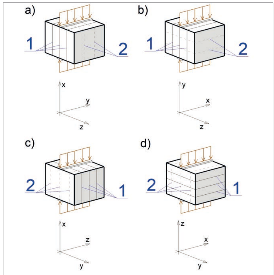
Rys. 5. Schemat kierunków obciążenia w badaniu wytrzymałości na rozciąganie przy rozłupywaniu dla połączeń międzywarstwowych: a) obciążenie wzdłuż osi X – wariant 1, b) obciążenie wzdłuż osi Y – wariant 1, c) obciążenie wzdłuż osi Z – wariant 1, d) obciążenie wzdłuż osi Z – wariant 2 (1 – połączenie międzywarstwowe, 2 – połączenie międzypasmowe)
