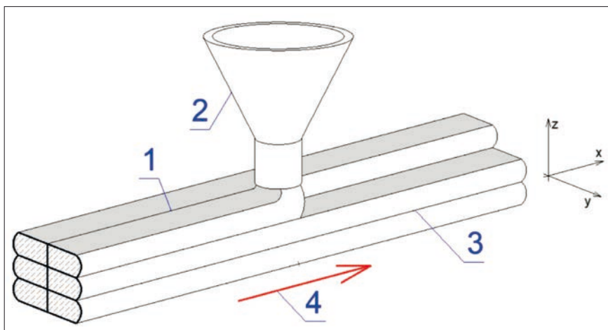
Rys. 1. Schematyczne przedstawienie procesu wydruku elementu wraz z osiami: 1) połączenie międzypasmowe, 2) głowica wraz z dyszą drukującą, 3) połączenie międzywarstwowe, 4) kierunek wydruku, X) kierunek ruchu głowicy drukującej, Y) kierunek międzypasmowy, Z) kierunek międzywarstwowy
