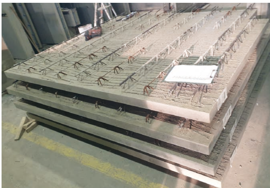
Fot. 1. Prefabrykowane stropy typu filigran
